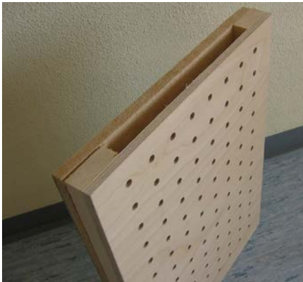
Bild 9: Photographische Aufnahme des Akustikelements (links) und Raumlufffeuchteauschläge im Testraum mit dem Akustikelement bezogen auf die Verhältnisse im Referenzraum (rechts)
